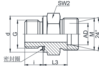
接头体
