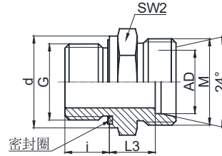
接头体
