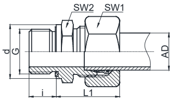
卡套式接头
