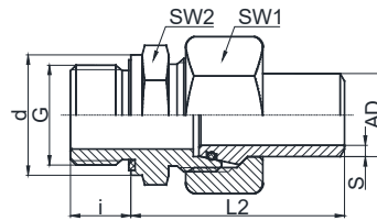
焊接式接头
