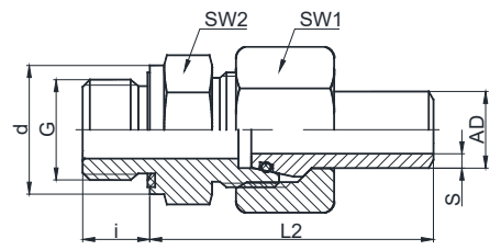
焊接式接头
