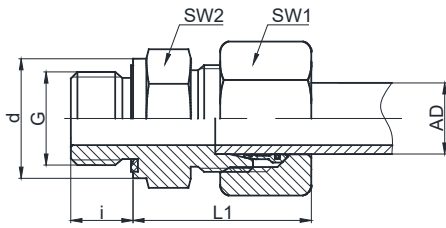
卡套式接头
